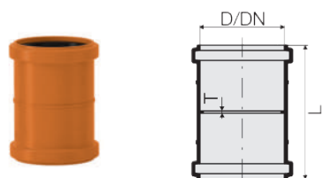
Manguito con tope
