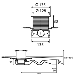
Sifón para plato de ducha extraplano T-58
