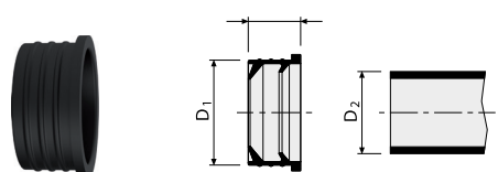
Adaptador elastomérico polivalente para conexión con otros sistemas
