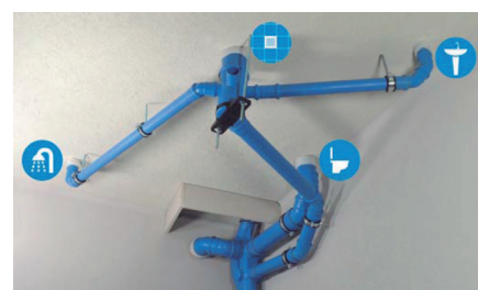
Sistema TRIPLUS
