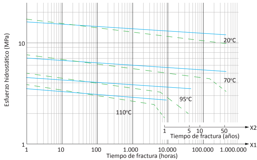
Comparación de las curvas de referencia para la resistencia esperada del PP-R (Tipo 3) y PP-R RP (Tipo 4)
