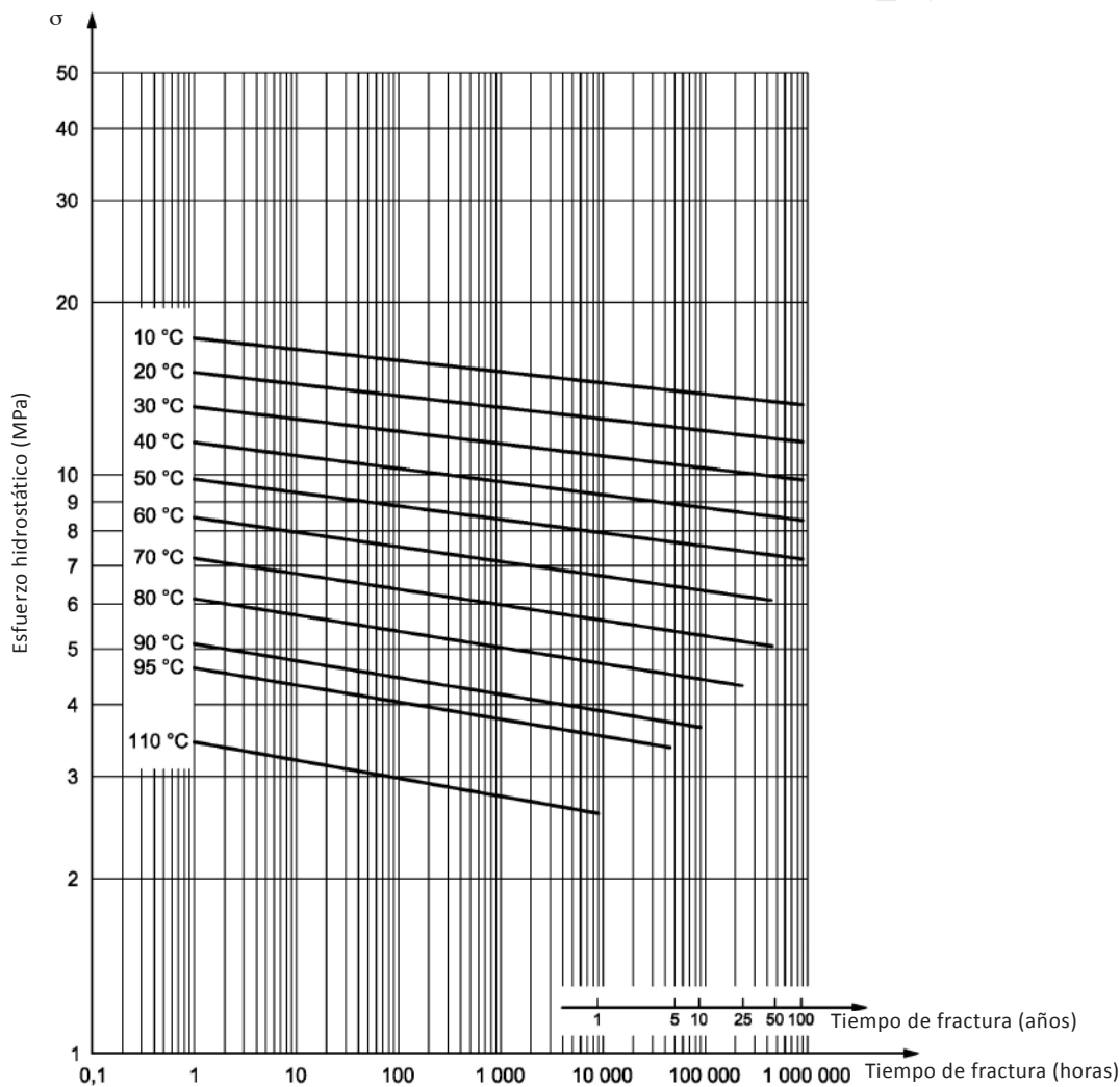
Curvas de referencia para la resistencia esperada del PP-R RP (Tipo 4) según NTP-ISO 15874
