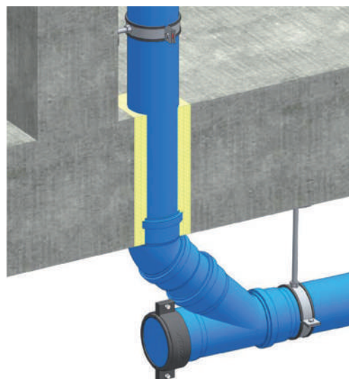
Ilustración 22 – Ejemplo de implementación de abrazadera/collar antideslizamiento.
