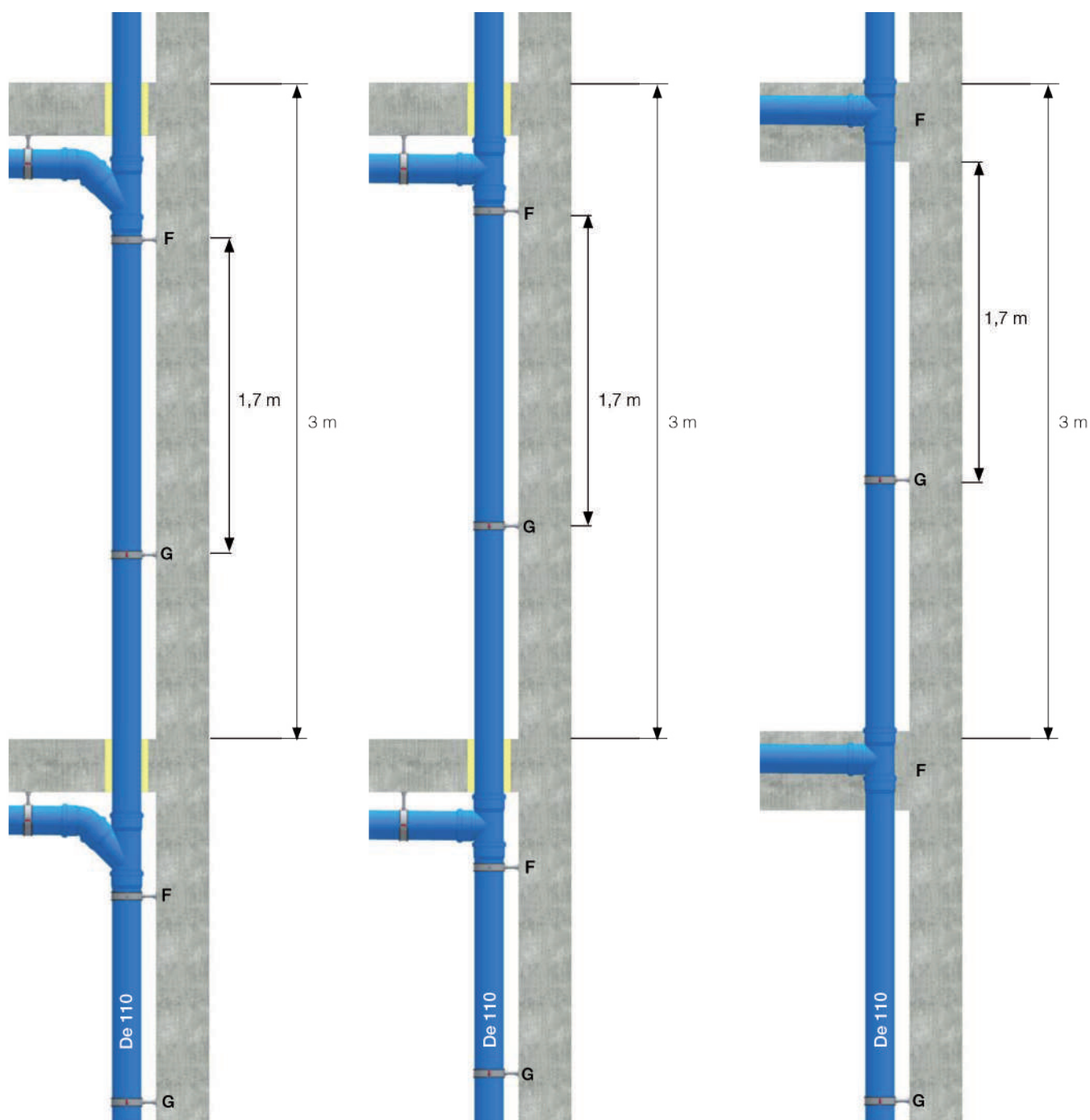
Ilustración 19 – Puntos de anclaje en tuberías verticales o sujeción en la colada de la tubería vertical.
