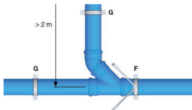
Ilustración 13 – Uso del sistema de sujeción adicional para cambios de dirección.
