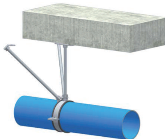
Ilustración 10 – Implementación de soporte triple
