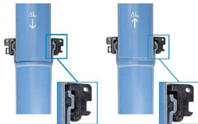
Ilustración 21 – Vista de sección de instalación de la abrazadera/collar antideslizamiento.
